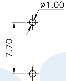
PCB Layout(Pattern Side)
