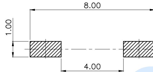
PCB Layout(Pattern Side)
